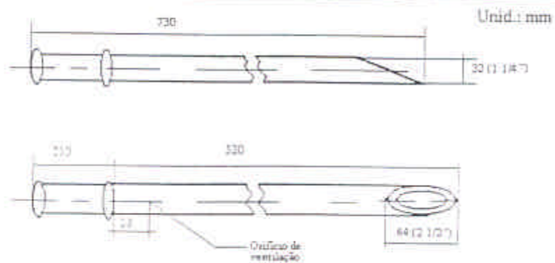
Figura 2 - Tubo amostrador para cimento em sacos
